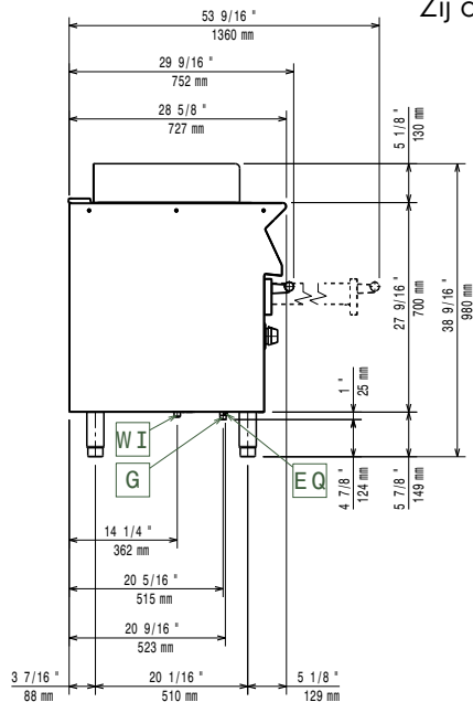
Zij aanzicht
